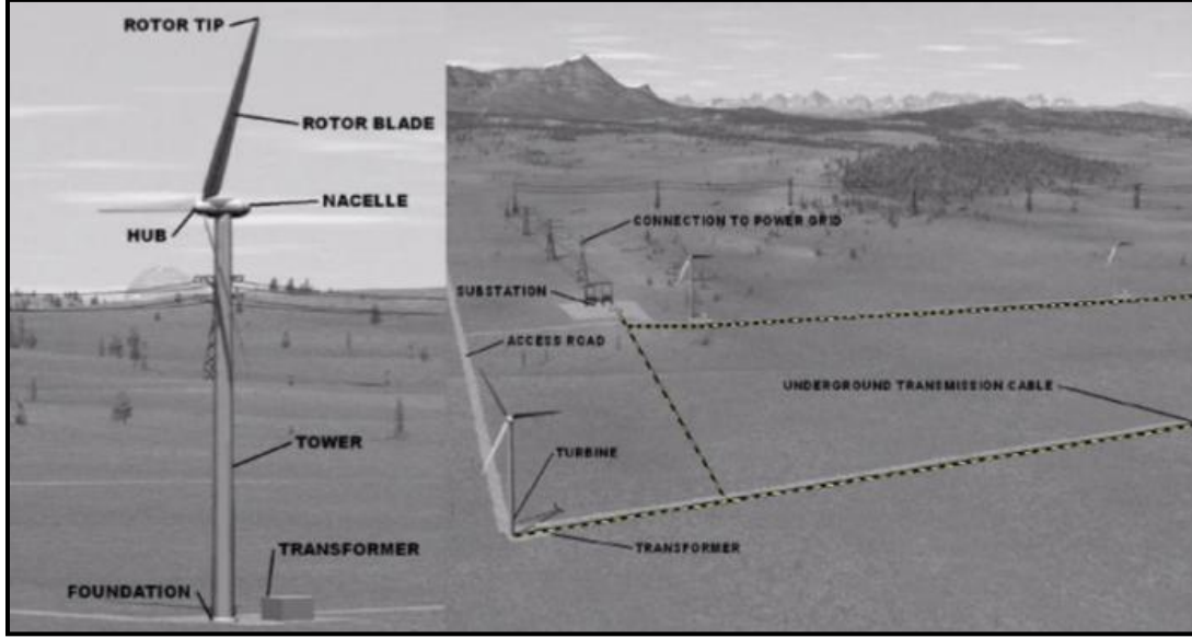
الشكل: 3 (أ) المكونات الهيكلية القياسية لتوربين الرياح. (ب) المكونات القياسية لمزرعة الرياح. (المصدر: إرشادات الصحة والسلامة والبيئة لطاقة الرياح، مؤسسة التمويل الدولية).
